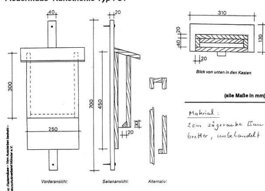
Fledermaus-Kunsthöhle Typ FS1
